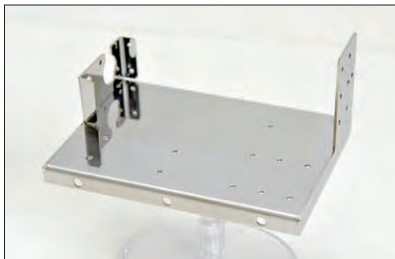
▲ベース (SUS,t=1.5)
