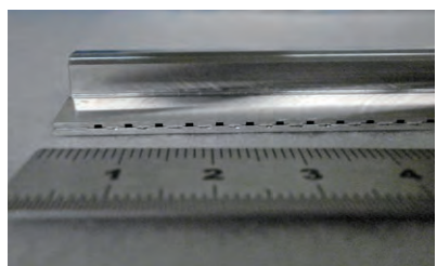
▲ブローノズル (側面) (ファイバーレーザータッパ溶接)
