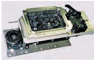
▲レーザーユニット (SUS,アルミ+黒アルミ)
