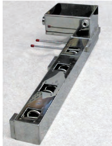
▲冷却板 (SUS,100×600)
